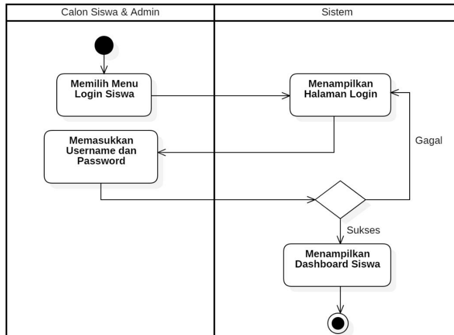
Gambar 4.4 Activity Diagram login oleh calon siswa dan admin
