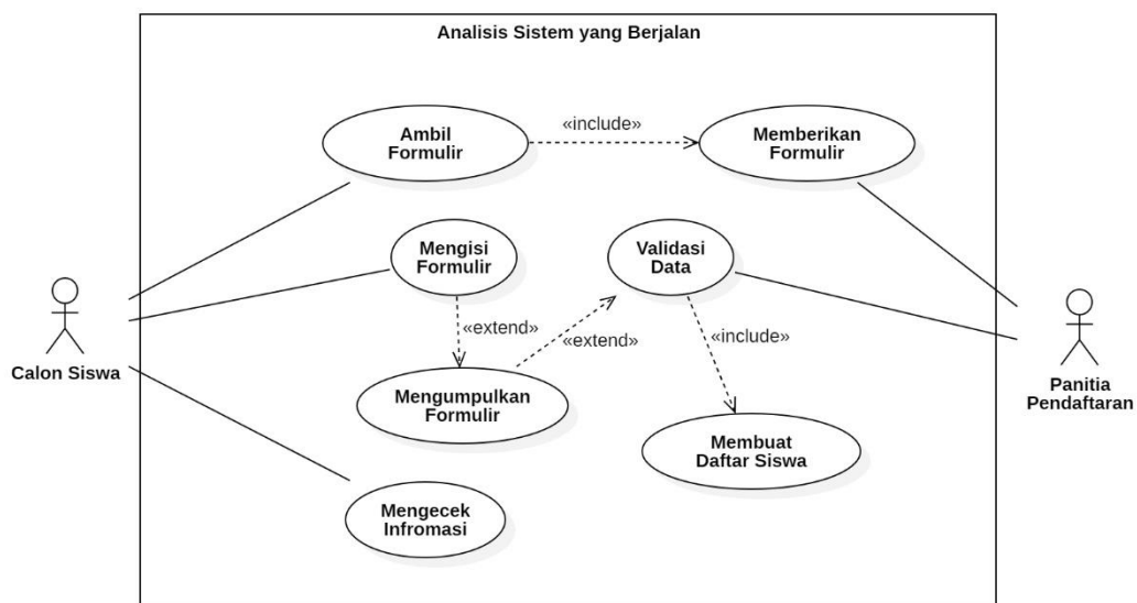
Gambar 4.1 Use Case Diagram yang sedang berjalan
