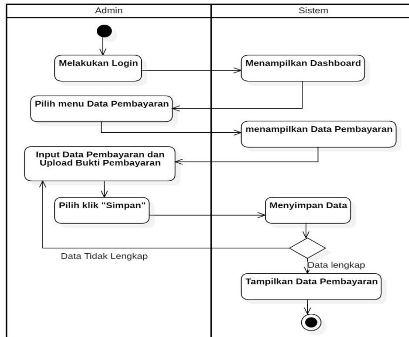
Gambar 4.10 Activity Diagram upload data pembayaran oleh admin
