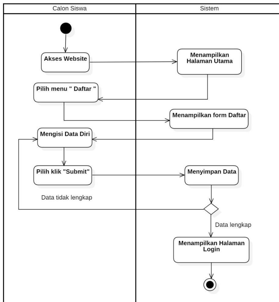
Gambar 4.3 Activity Diagram Daftar dan mengisi Formulir oleh Calon Siswa
