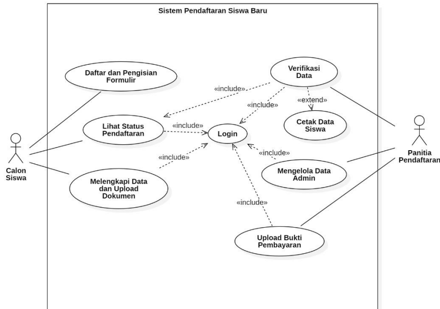
Gambar 4.2 Use Case Diagram Sistem yang diusulkan
