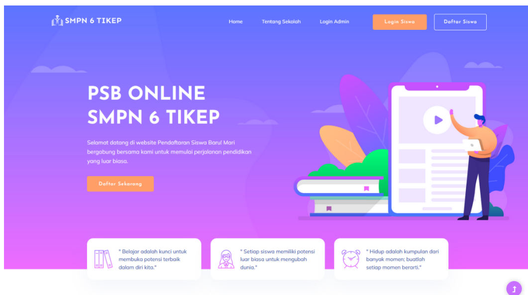
Gambar 4.12 Tampilan Beranda
