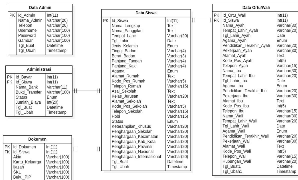
Gambar 4.11 Relasi Tabel
