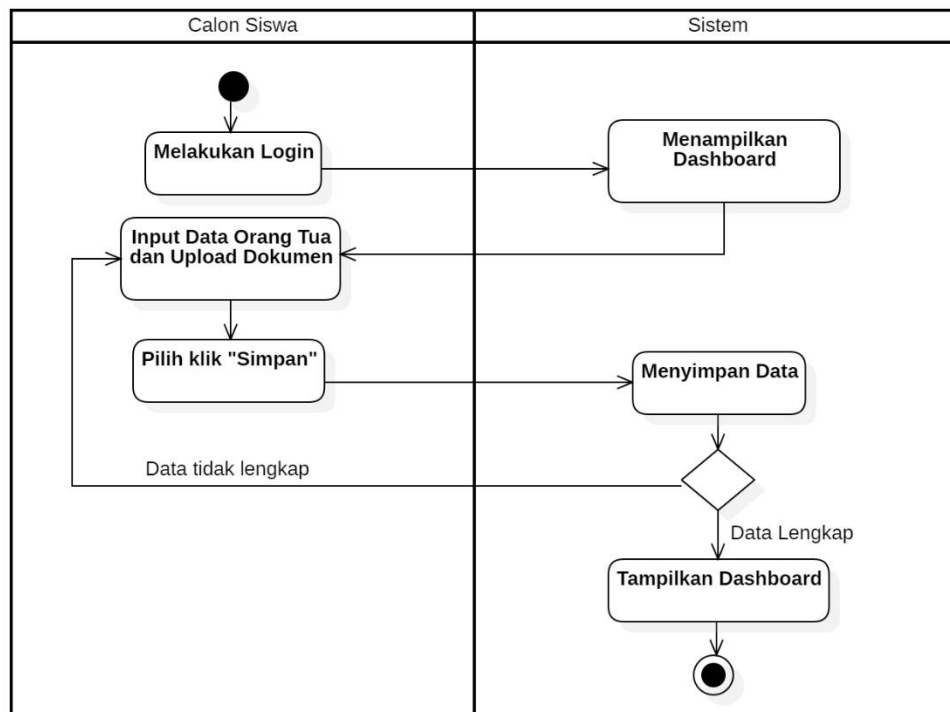
Gambar 4.6 Activity Diagram Lengkapi data dan upload dokumen oleh calon siswa
