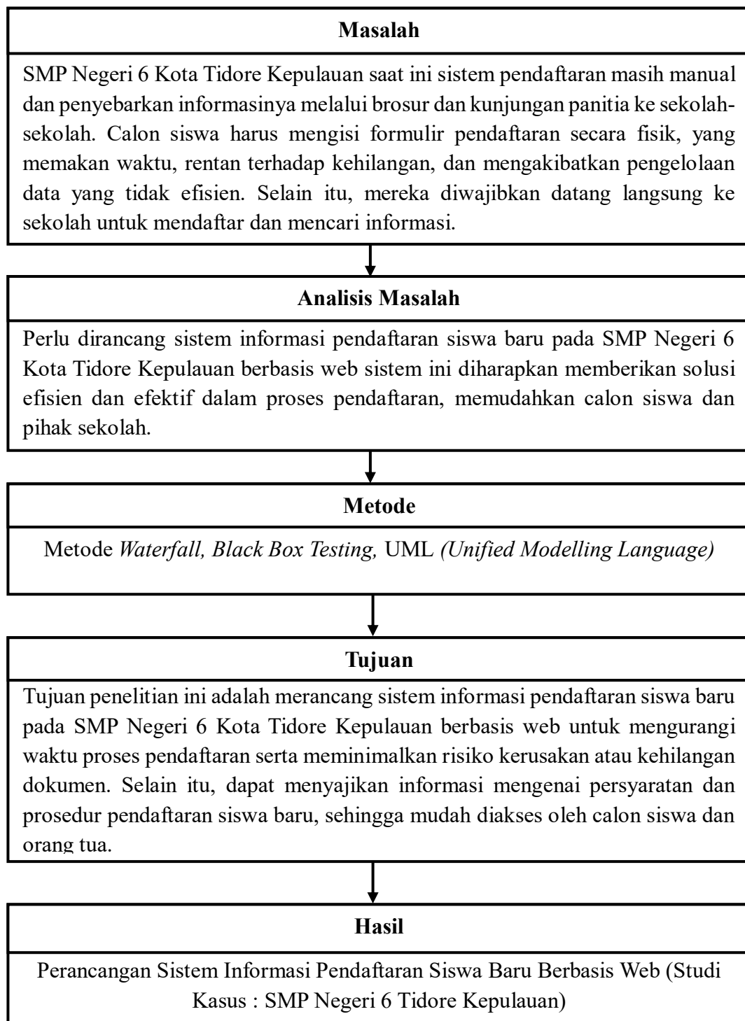
Gambar 2.2 Kerangka Berpikir
