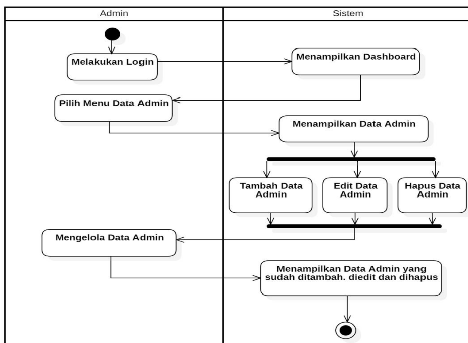
Gambar 4.9 Activity Diagram mengelola data admin oleh admin
