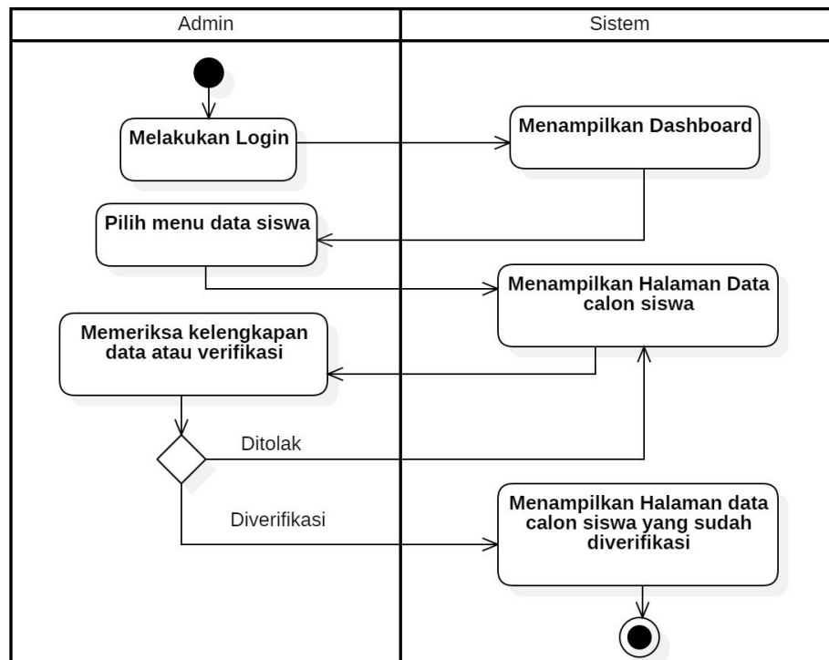
Gambar 4.8 Activity Diagram verifikasi data siswa oleh admin
