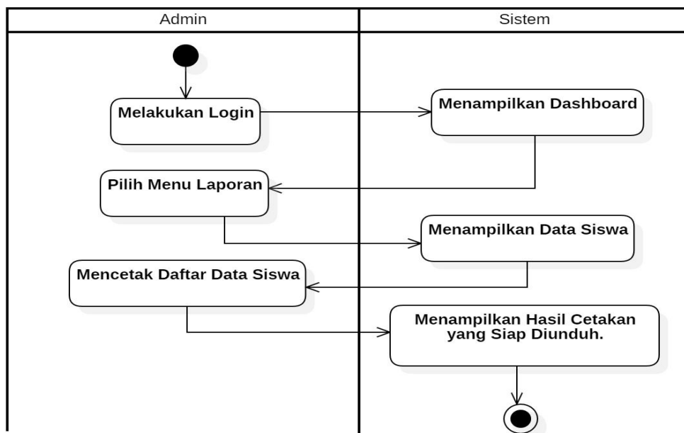
Gambar 4.5 Activity Diagram mencetak daftar siswa oleh admin
